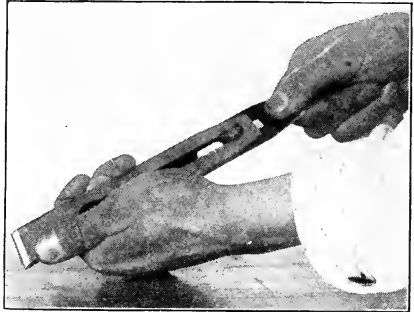
Fig. 106—Sliding Cap Iron
